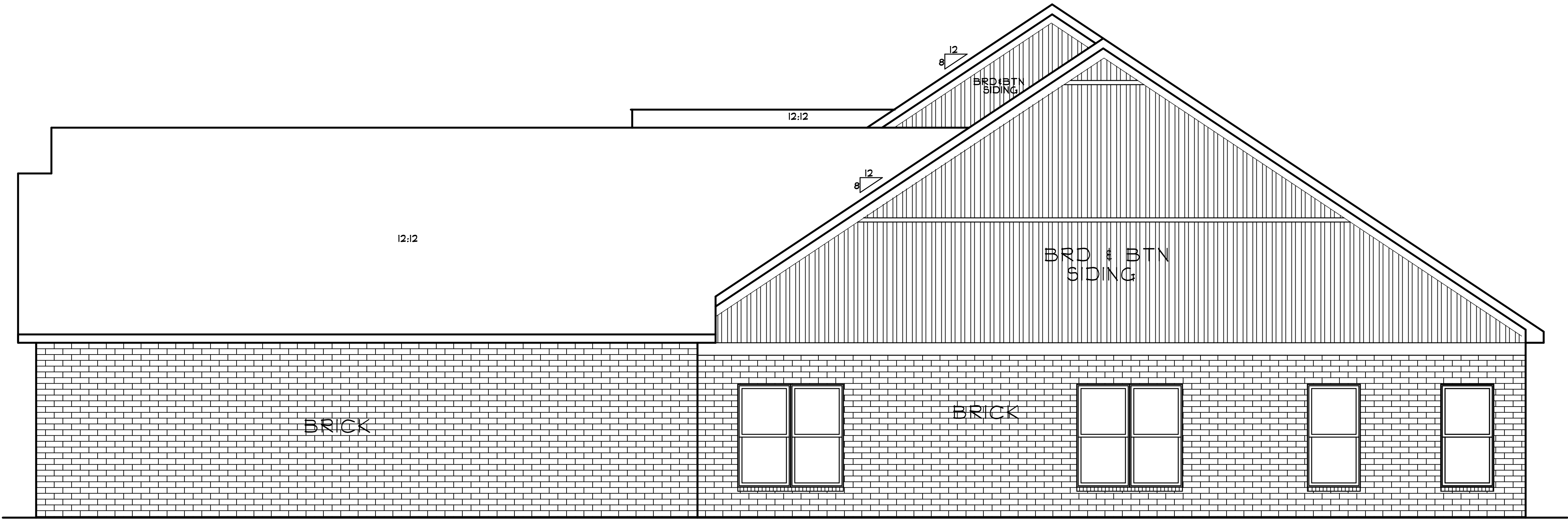
RIGHT ELEVATION
